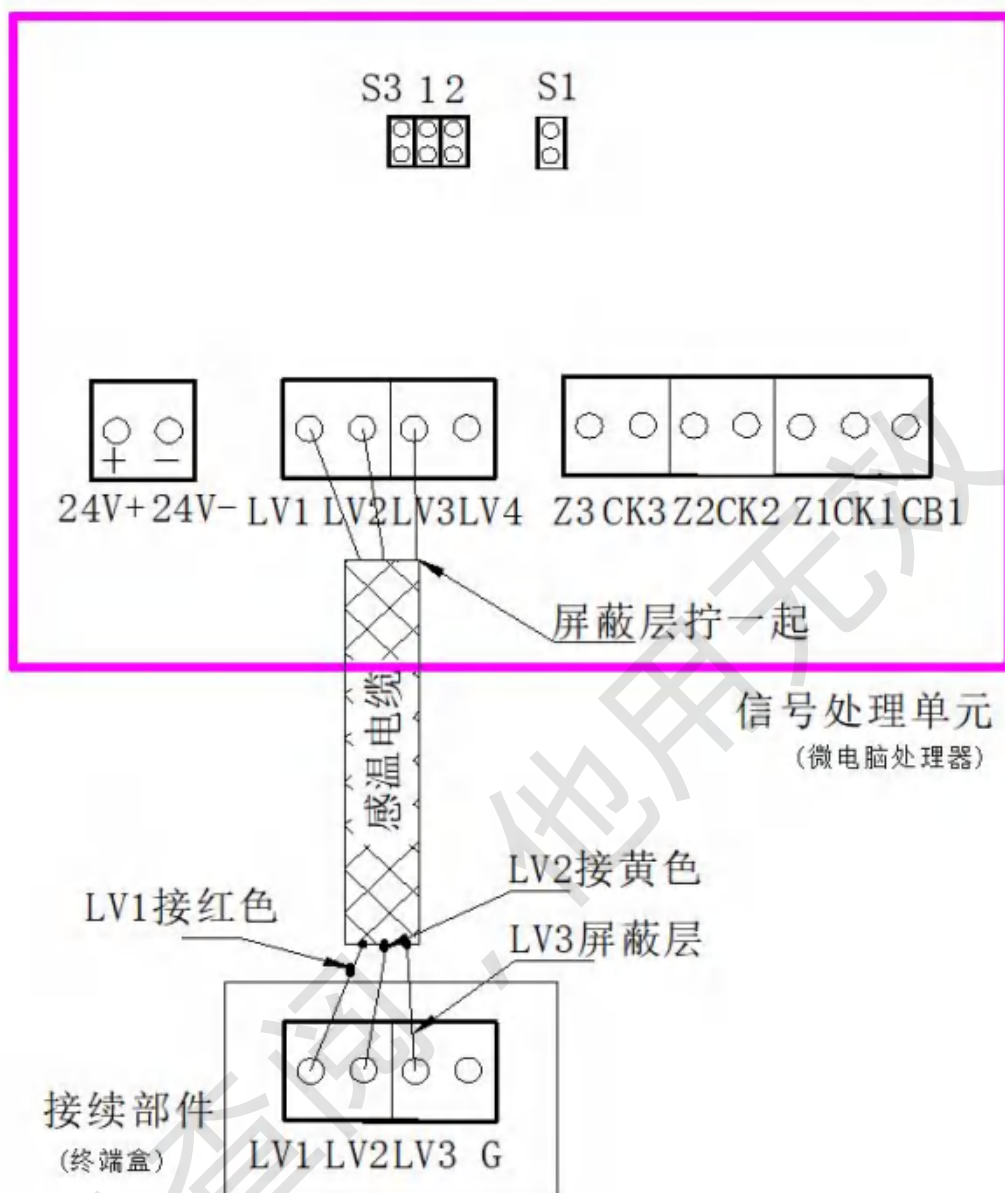
图4 探测器应用系统图
