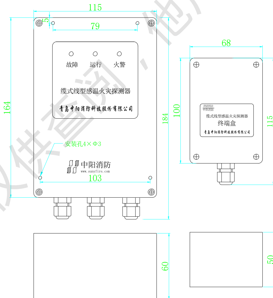
图 1 微电脑处理器和终端盒外形示意图 单位：mm
